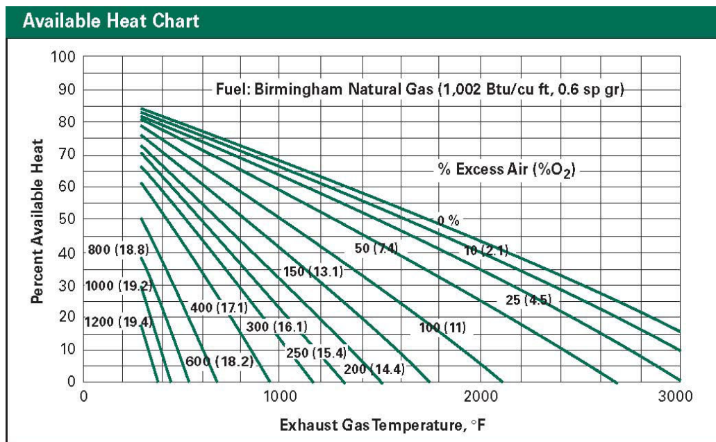
Rys.1 Diagram publikowany w materiałach firmy Super Systems INC, USA
